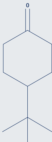
4-t-butylcyclohexanone
